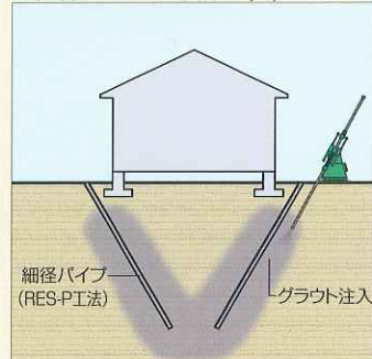
グラウトと細径パイプを用いた斜杭・組杭を併用して、地盤の沈下を防止。
