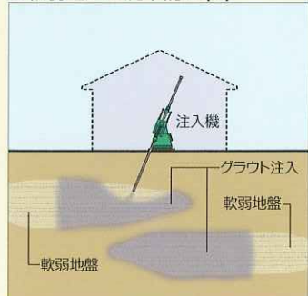
地盤中に軟弱層などがあり、地盤の支持力が弱い場合、グラウトを注入して地盤の沈下を防止。
