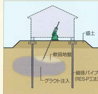
軟弱な地盤に盛土をした場合、地盤改良工事を施工しても圧密沈下を起こし易いため、グラウトを注入して地盤の沈下を防止。
