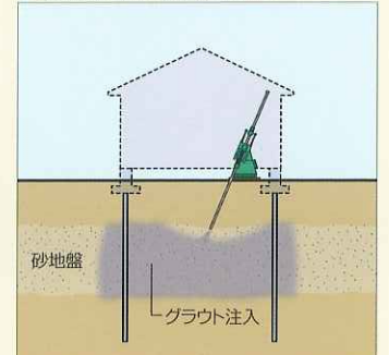
地盤中に砂層がある場合、地震の際に液状化現象を起こしやすいため、グラウトを注入して液状化を防止。
