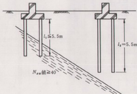
図-3 採用できない地盤
