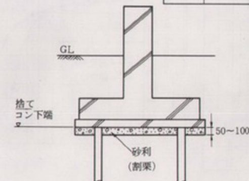
図-4 基礎本体と鋼管頭部との関係
