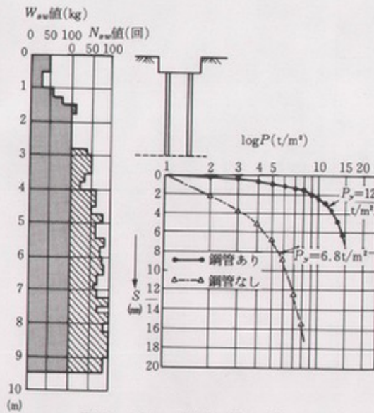
図-8 P-log S関係 (その3)
