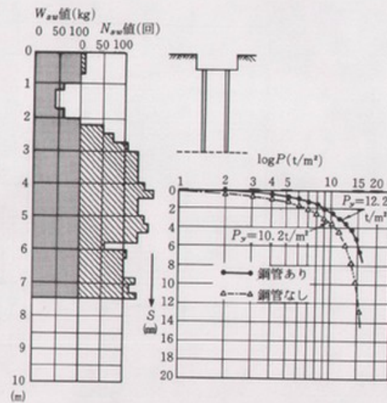
図-9 P-log S関係 (その4)
