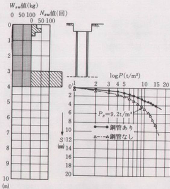
図-10 P-log S関係 (その5)
