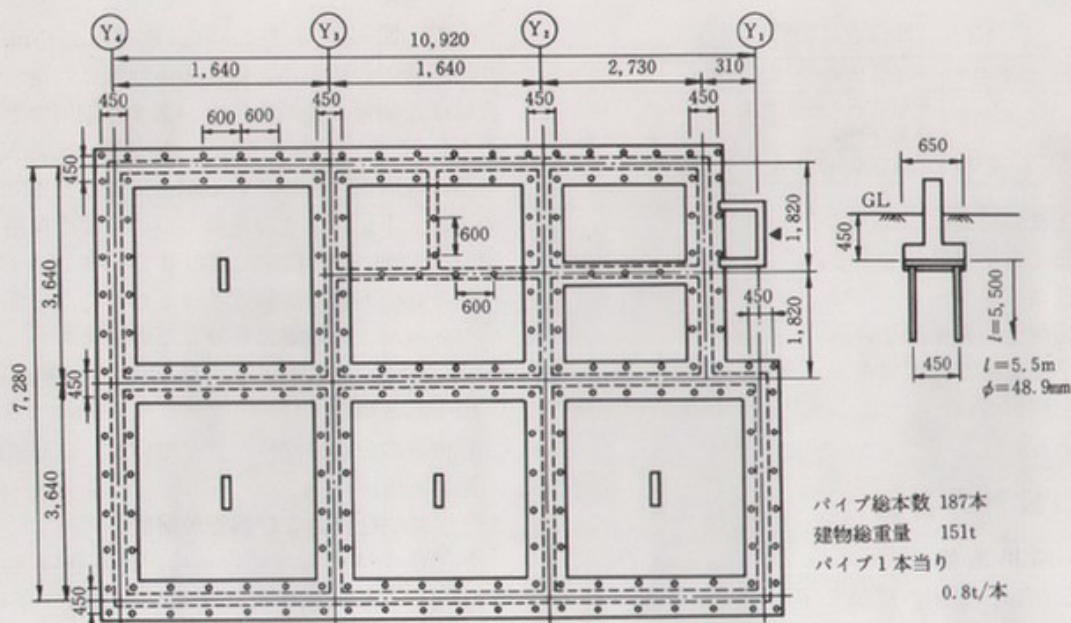
図-5 鋼管の配置例
